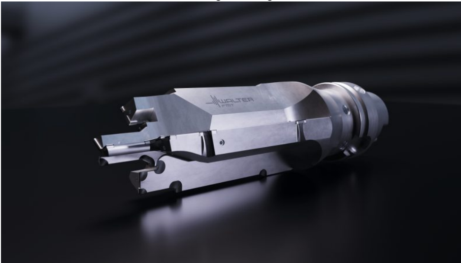
Beispiel für ein individuelles Werkzeug für die Leichtbauzerspanung (Bild: Walter).
